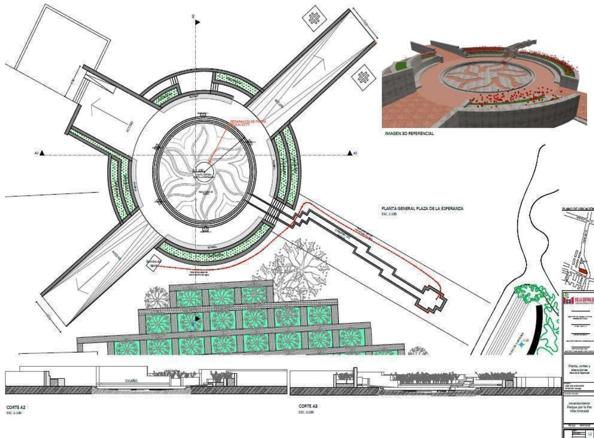
Plano de la intervención propuesta, recupera la recirculación de agua y modifica la red de alimentación para evitar el efecto de las raíces del Ombú
